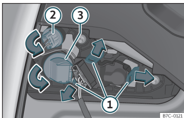
Afb. 50 Fitting uitbouwen.
