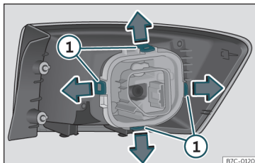
Afb. 48 Bevestigingslappen aan de achterzijde van het achterlicht.
