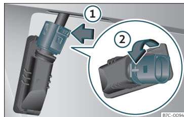
Afb. 52 Kentekenplaatverlichting: fitting uitbouwen.
